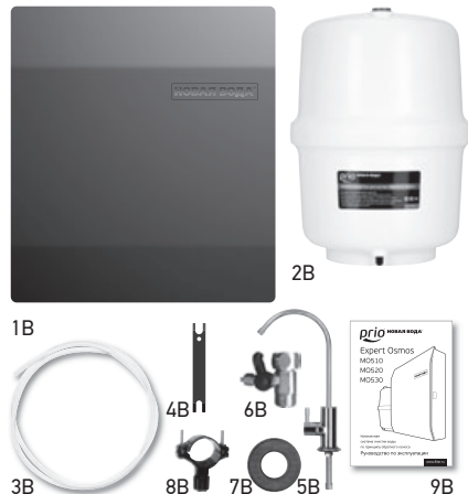
Рис. 3. Комплектация фильтра Expert Osmos.
